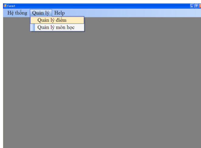
Hình 9. 44. Form frmMain
