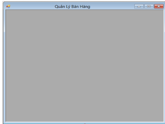
Hình 9. 20. Form frmMain
