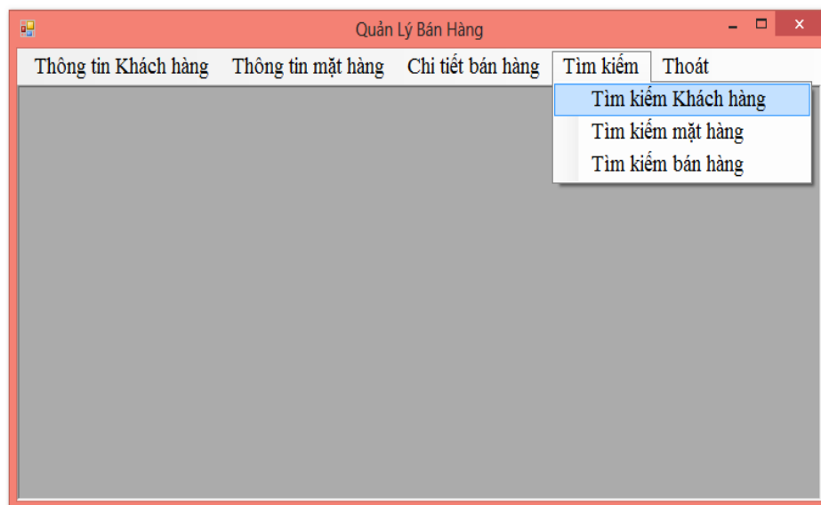
Hình 9.7. Form MDI
