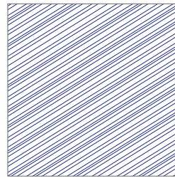
\nu_2/\nu_1 = (\sqrt{5} - 1)/2 : dense
