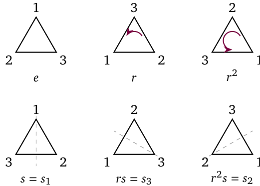
1.4 pav.: Trikampio simetrijos operacijos. Skaičius kampuose nurodo, kuri pradinė viršūnė ten atsiduria. Viršuje – posūkiai, apačioje – atspindžiai su punktyrinėmis ašimis.
