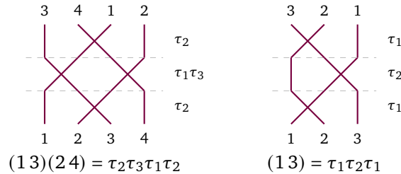
1.3 pav.: Perstatymas kaip virvučių pynė, skaitoma iš apačios į viršų ir suverta iš elementarių sluoksnių. Nesusikertantys sluoksniai, kaip \tau_1 ir \tau_3 , braižomi viename lygyje.
