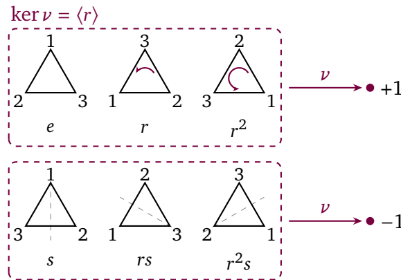
2.1 pav.: Orientacijos homomorfizmas \nu: D_3 \rightarrow \{\pm 1\} . Visi trys posūkliai (viršuje) pereina į +1 , visi trys atspindžiai (apačioje) – į -1 : kiekvienas brūkšninis blokas suspaudžiamas į vieną tašką, o viršutinis blokas yra branduolys. Per izomorfizmą D_3 \cong S_3 tai yra ženklas \text{sgn} : posūkliai yra lyginiai perstatymai, atspindžiai – nelyginiai.
