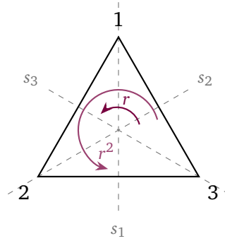
1.1 pav.: Šešios lygiakraščio trikampio simetrijos operacijos: neutralusis elementas, du posūkiai apie centrą ir atspindžiai trijų pusiaukraštinių atžvilgiu. Ašis s_i eina per viršūnę i .
