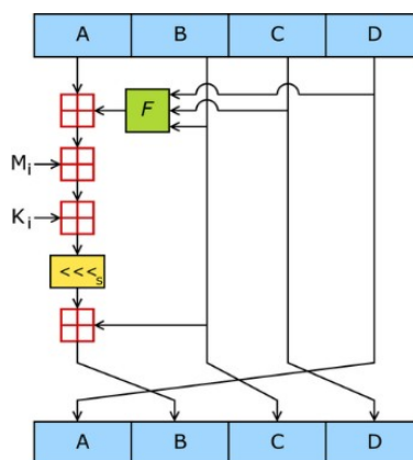
Hình ảnh 4: Giải thuật MD5
