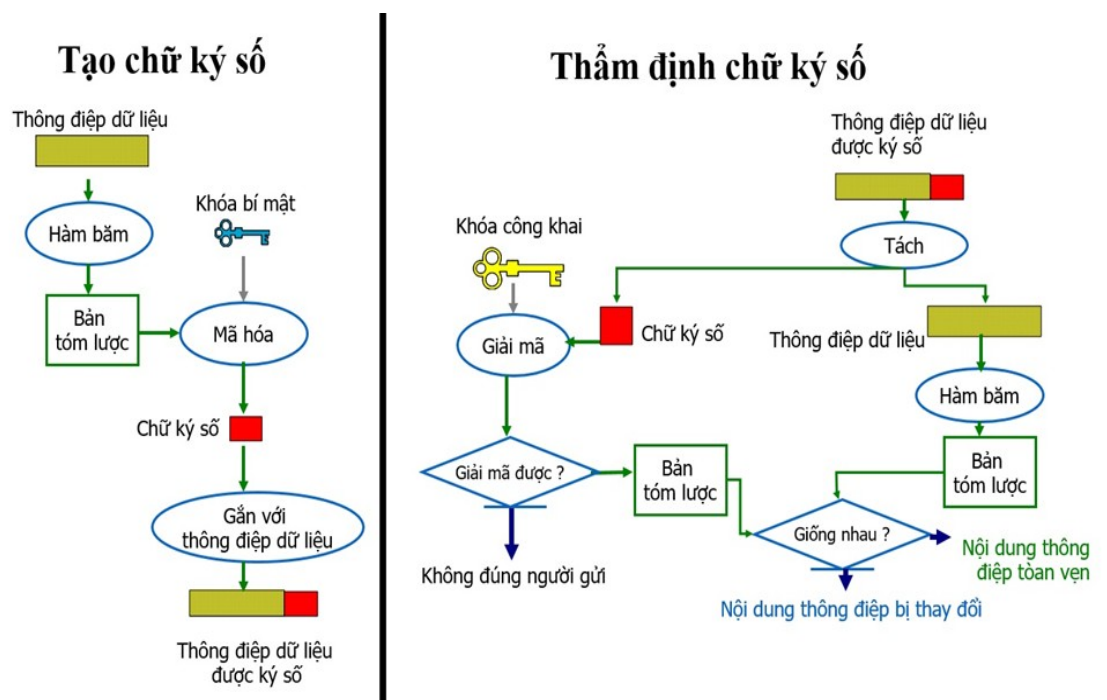
Hình ảnh 7: Chức năng tạo chữ ký số và thẩm định chữ ký số
