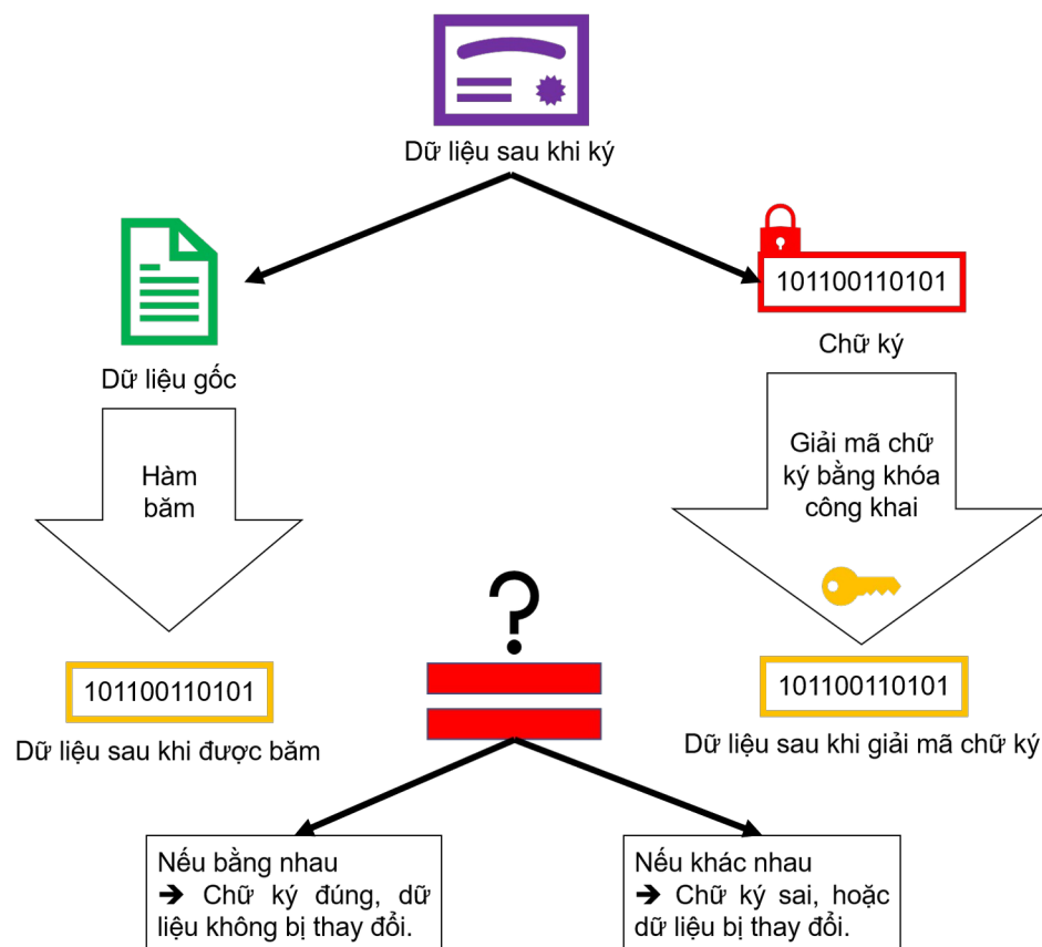
Hình ảnh 2: Quá trình kiểm tra chữ ký
