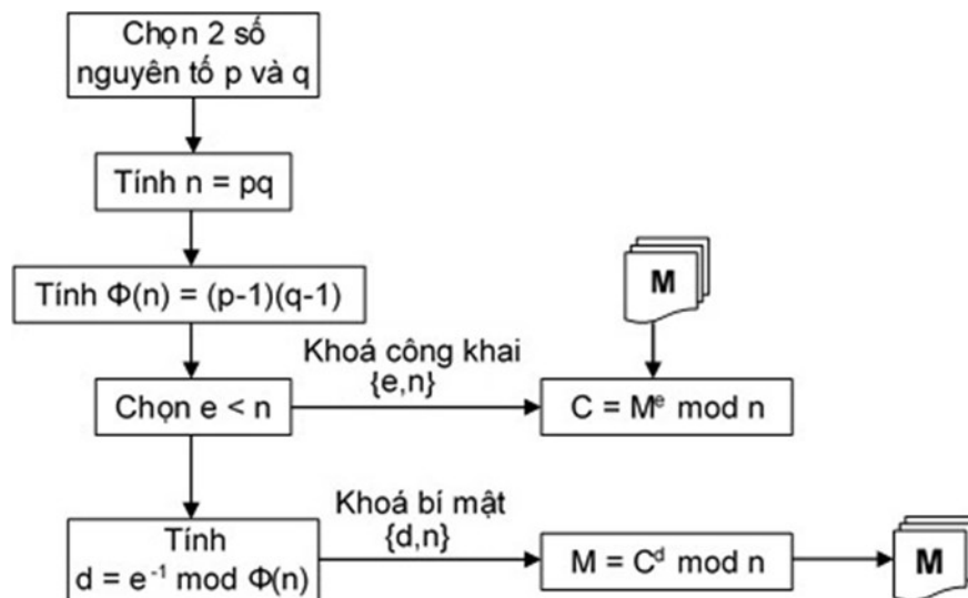
Hình ảnh 2 Sơ đồ biểu hiện RSA mã hóa thuật toán.
