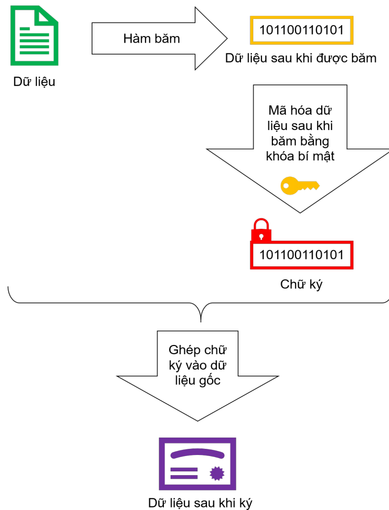
Hình ảnh 1: Quá trình tạo chữ ký
