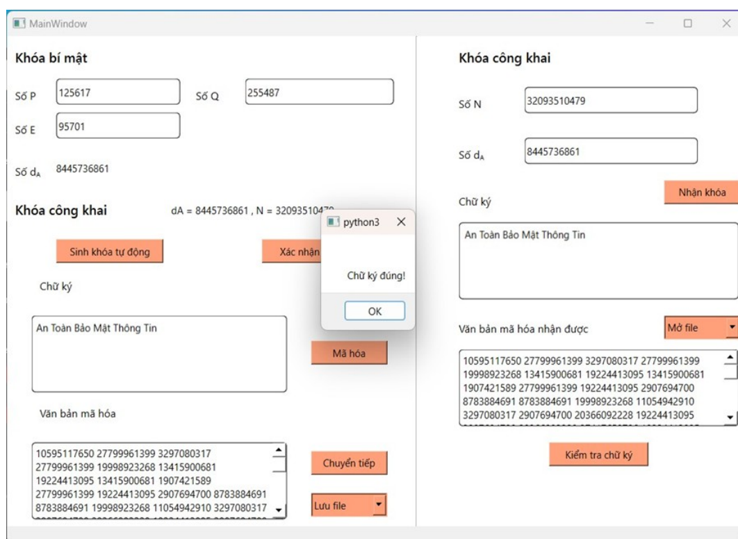
Hình ảnh 16: Kết quả đúng sau khi mã hóa chữ ký
