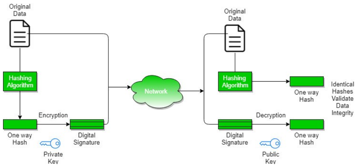
Hình ảnh 5: Sơ đồ hệ thống chữ ký số RSA
