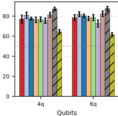
EuroSAT
