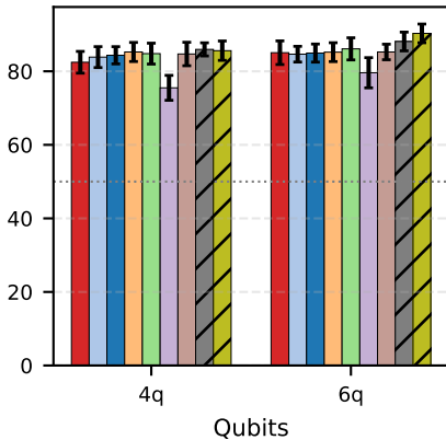
MNIST
