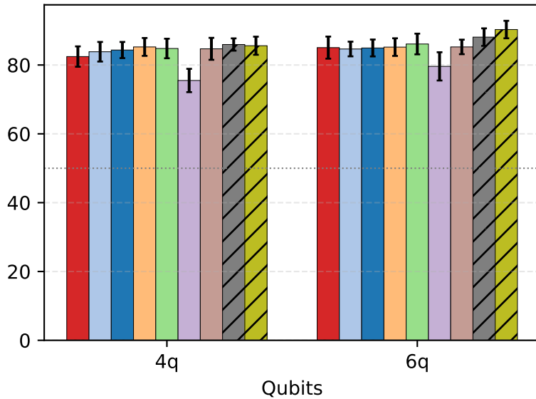
MNIST
