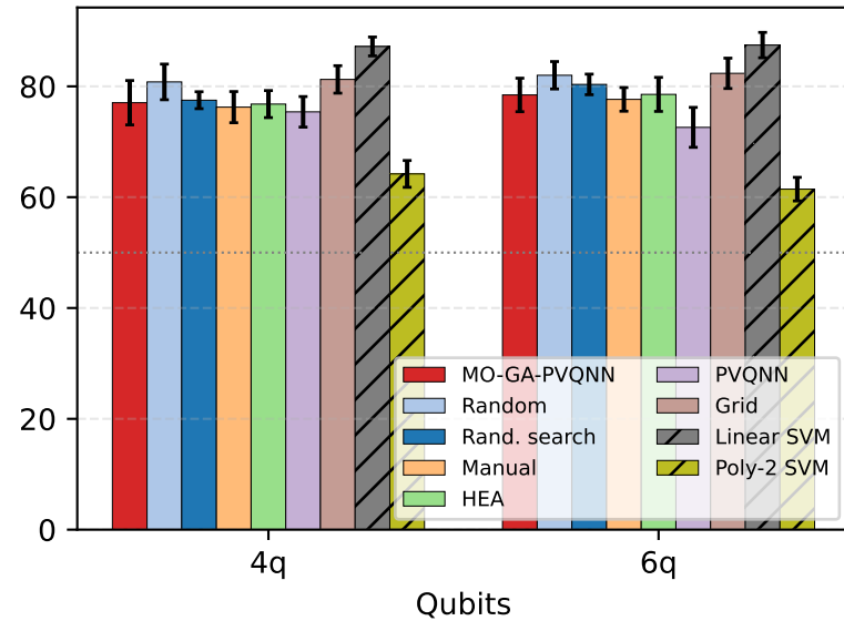
EuroSAT
