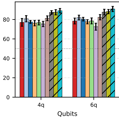
EuroSAT
