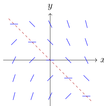
Example 2: y' = -x - y
