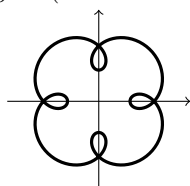
Epitrochoid
