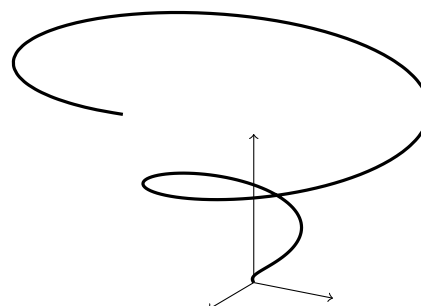
Cone
