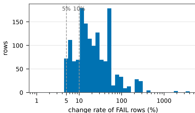
図 4 全 FAIL 行 (1,465 行) の変動率分布 (対数軸). 破線は既定閾値 (detection 5% / db 10%). 閾値近傍の 5 から 20%帯に対し, 100%超の構造イベント群が裾として分離する. FAIL 行のみを重複 (cron 再実行) 込みで集計した分布であり, 全更新の変動率分布ではない.
