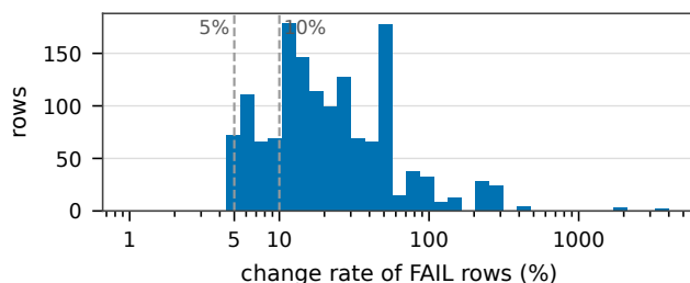
図 4 FAIL した 1,465 行の変動率分布 (対数軸)。5-20% の帯に対し、100% を超える構造的イベントが裾を形成する。cron による重複を含み、閾値未満の更新を含まない。
