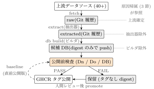
図 1 脆弱性 DB 公開パイプラインと公開前検査。全工程が Git 履 歴管理 [2] され、原因帰属 (3 節) は各工程の履歴を参照する。
