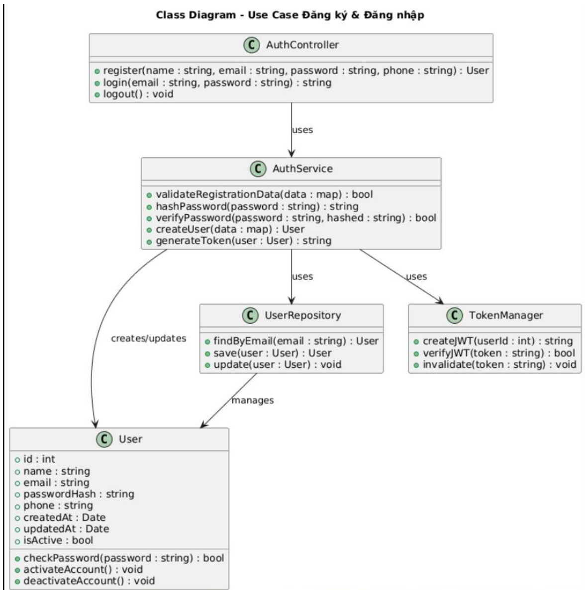
Hình 28: Biểu đồ class cho use case đăng ký và đăng nhập
