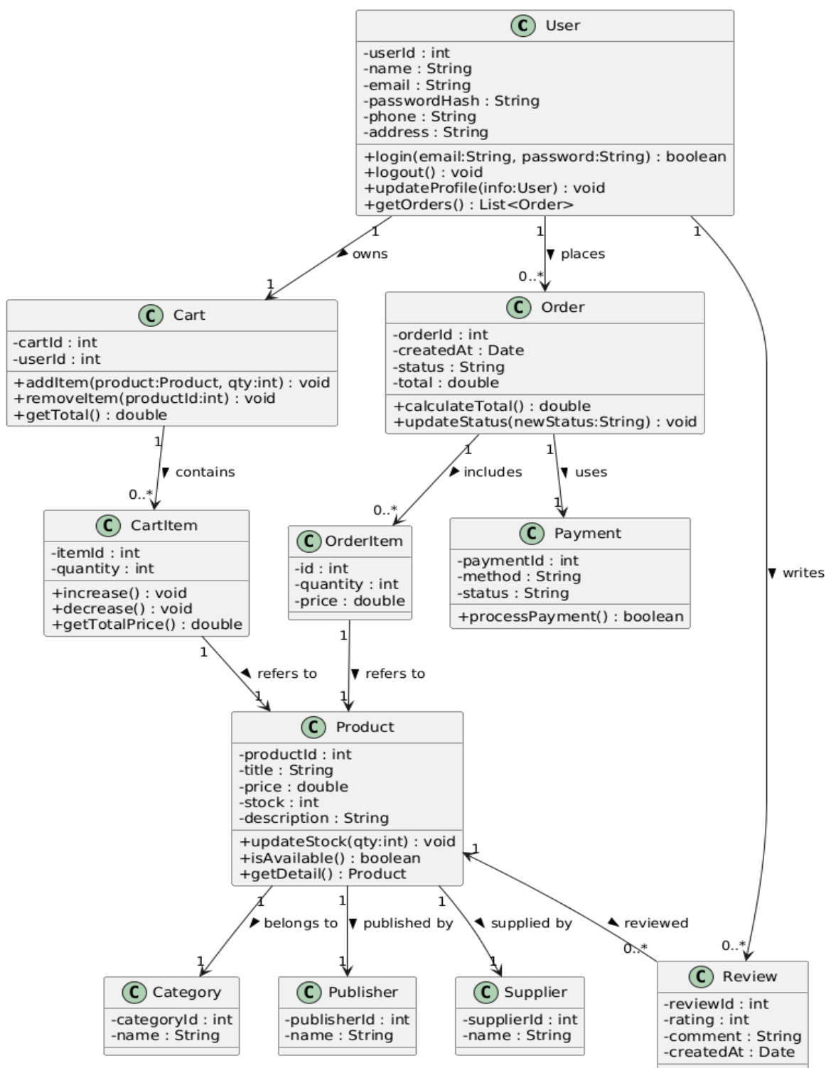
Hình 27: Biểu đồ class Tổng Quan cho các lớp quan trọng
