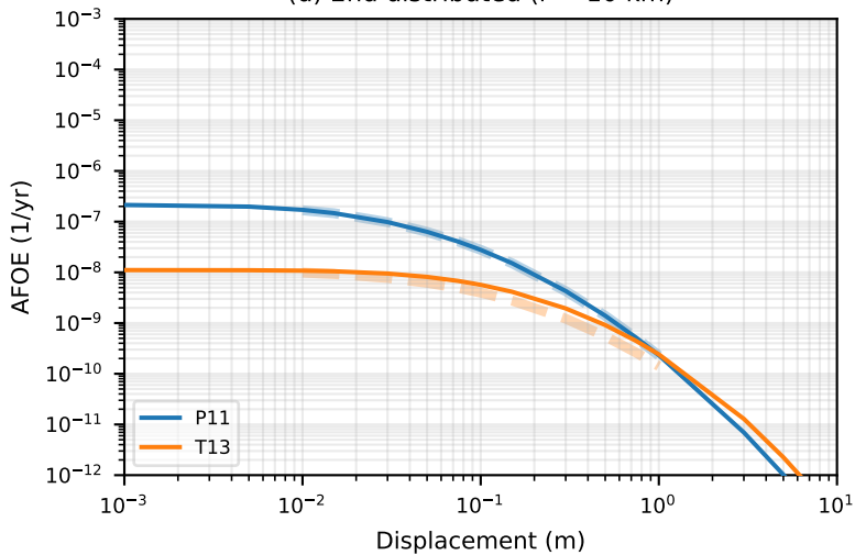
(d) 2nd distributed ( r = 10 km)
