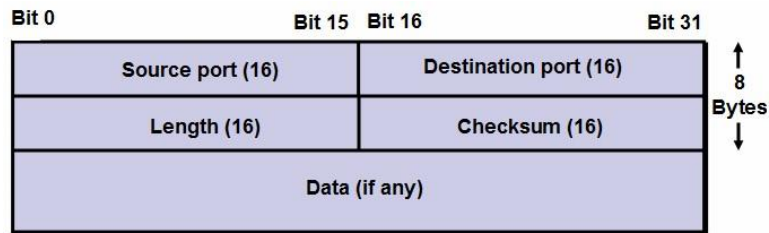
Hình 2.17. Khuôn dạng UDP Datagram
