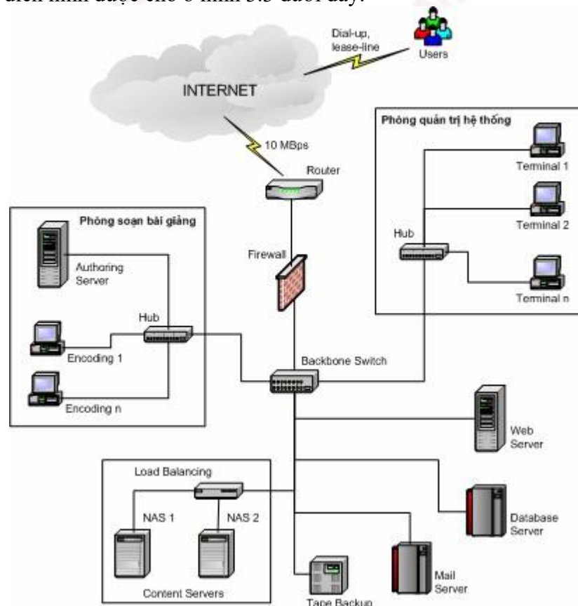
Hình 3.3: Mô hình mạng trung tâm cho hệ thống e-learning
