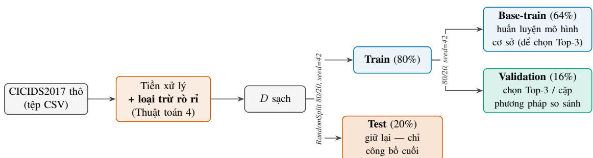
Hình 3.2. Sơ đồ phân chia dữ liệu CICIDS2017: chia 80/20 thành train/test ( seed=42 ); tập train tách tiếp 80/20 thành base-train và validation phục vụ chọn lọc, tập test được giữ lại chỉ để công bố kết quả cuối
