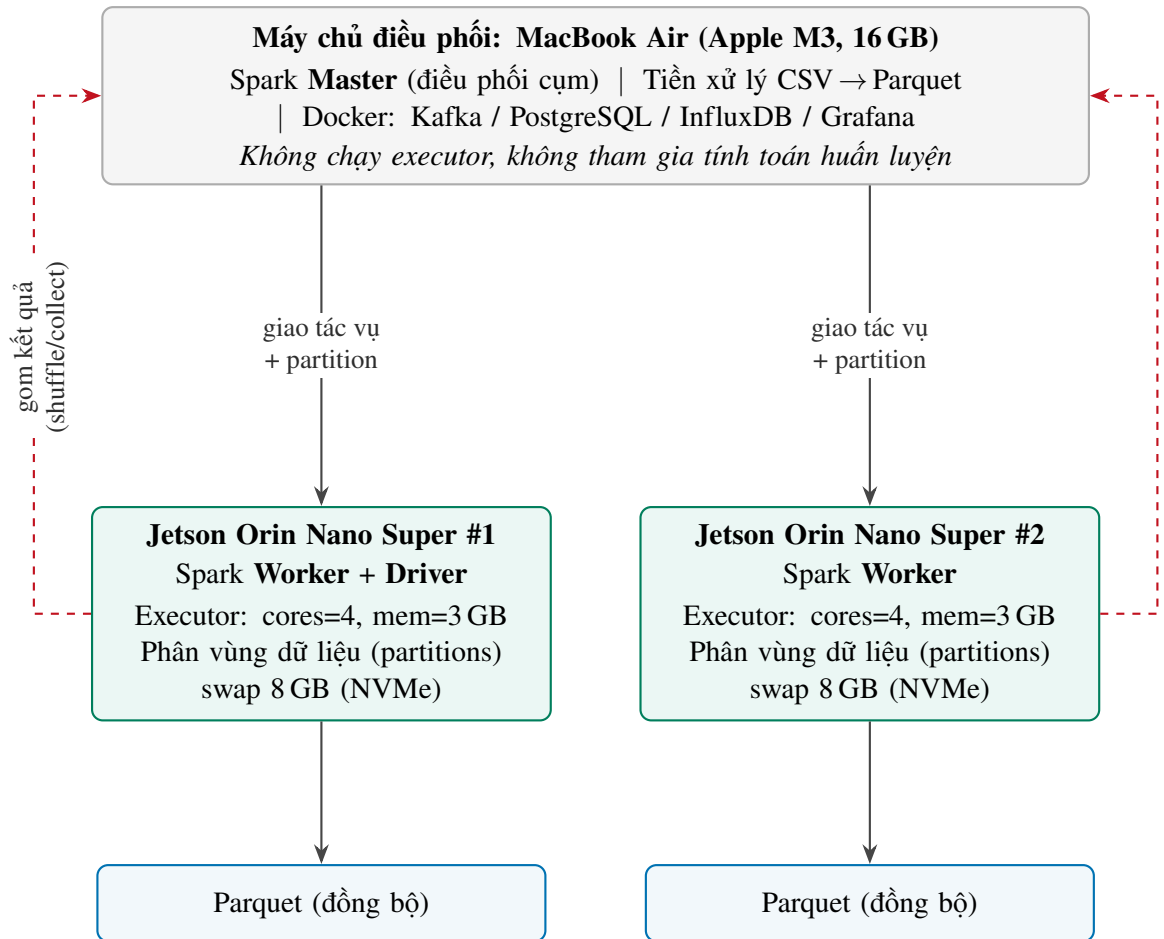
Hình 4.1. Cụm huấn luyện phân tán Apache Spark Standalone: máy chủ điều phối (master) và hai Jetson worker/executor
