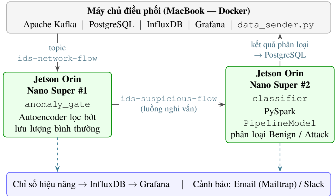
Hình 4.5. Kiến trúc hệ thống phát hiện xâm nhập phân tán thời gian thực trên cụm 2 Jetson Orin Nano Super
