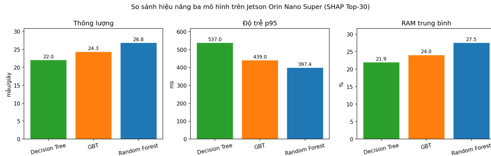
Hình 4.12. So sánh hiệu năng ba mô hình trên Jetson Orin Nano Super
