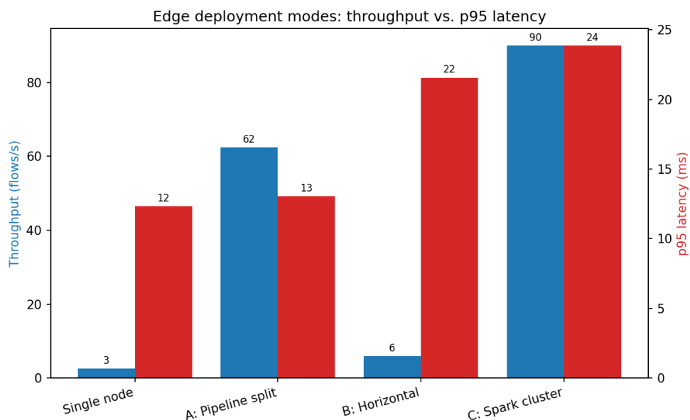
Hình 4.11. Thông lượng và độ trễ p95 của bốn chế độ triển khai trên cụm 2 Jetson
