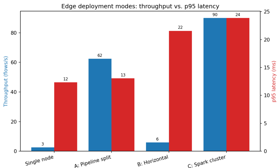
Hình 4.12. Thông lượng và độ trễ p95 của bốn chế độ triển khai trên cụm 2 Jetson
