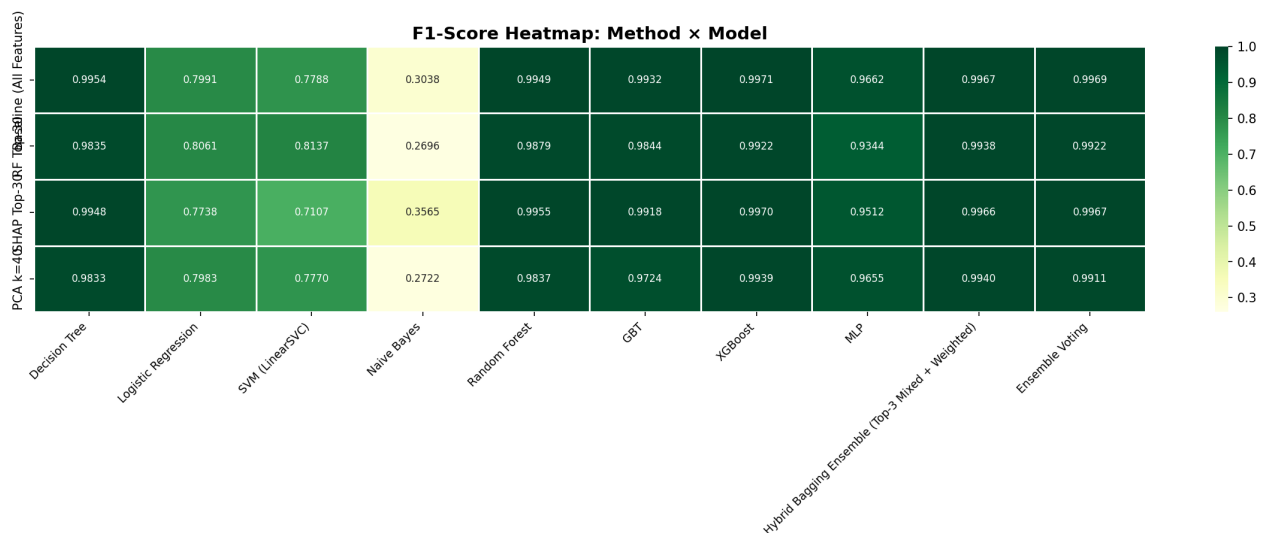
Hình 3. Heatmap F1 theo phương pháp và thuật toán (nhị phân, đã loại cổng).
