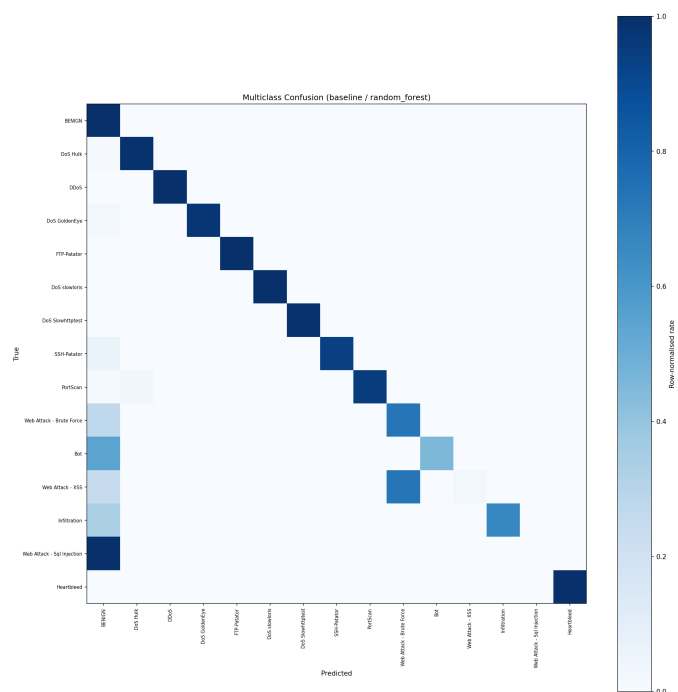
Hình 5. Ma trận nhầm lẫn đa lớp (chuẩn hoá theo hàng).
