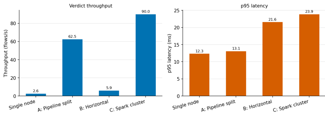
Hình 4.12. Thũng lng vị tr p95 ca bn cu hnh (mt nút c s + ba ch phón tòn) trón cm 2 Jetson
