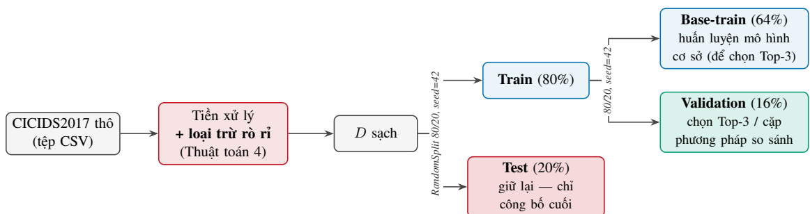
Hình 3.2. Sơ đồ phân chia dữ liệu CICIDS2017 (train/test 80/20, seed=42 ; train tách tiếp 80/20 thành base-train/validation)
