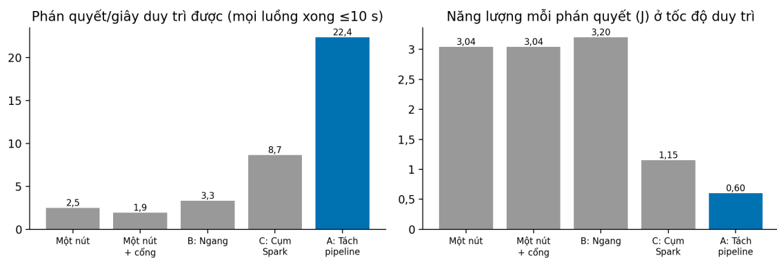
Hình 4.13. Năng lực duy trì (trái) và năng lượng mỗi phán quyết ở tốc độ duy trì (phải) của năm cấu hình triển khai trên cụm 2 Jetson
