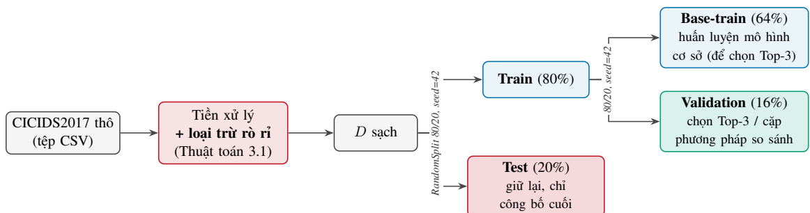
Hình 3.2. Sơ đồ phân chia dữ liệu CICIDS2017 (train/test 80/20, \text{seed}=42 , trong đó train tách tiếp 80/20 thành base-train/validation)
