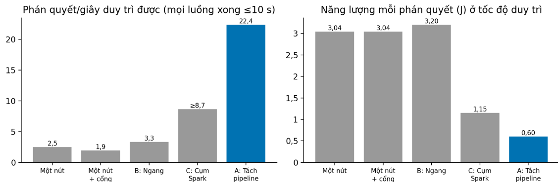
Hình 4.15. Năng lực duy trì (trái) và năng lượng mỗi phán quyết ở tốc độ duy trì (phải) của năm cấu hình triển khai trên cụm 2 Jetson. Cột của cụm Spark là cận dưới, cột một nút + cổng xem chú thích Bảng 4.19
