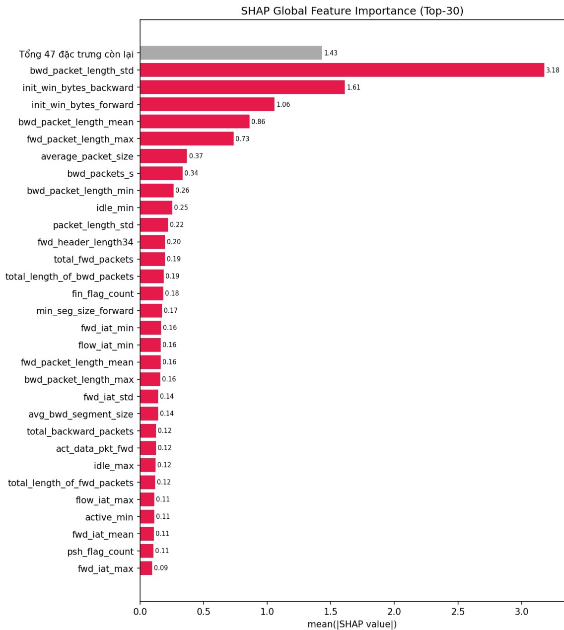
Hình 4.2. Top 30 đặc trưng quan trọng theo giá trị trung bình tuyệt đối SHAP của mô hình XGBoost
