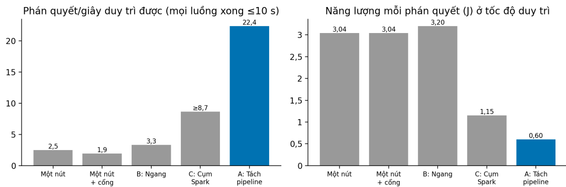
Hình 4.13. Năng lực duy trì (trái) và năng lượng mỗi phán quyết ở tốc độ duy trì (phải) của năm cấu hình triển khai trên cụm 2 Jetson. Cột của cụm Spark là cận dưới, cột một nút + cổng xem chú thích Bảng 4.19
