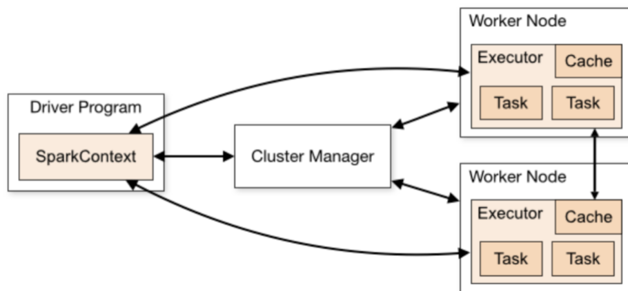
Hình 2.3. Sơ đồ kiến trúc hệ thống Apache Spark [25]
