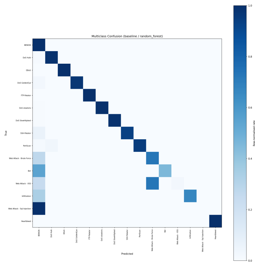
Hình 4.4. Ma trận nhầm lẫn đa lớp theo loại tấn công (chuẩn hoá theo hàng)
