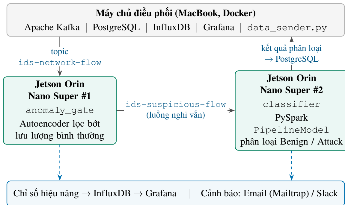
Hình 4.5. Kiến trúc hệ thống phát hiện xâm nhập phân tán thời gian thực trên cụm 2 Jetson Orin Nano Super
