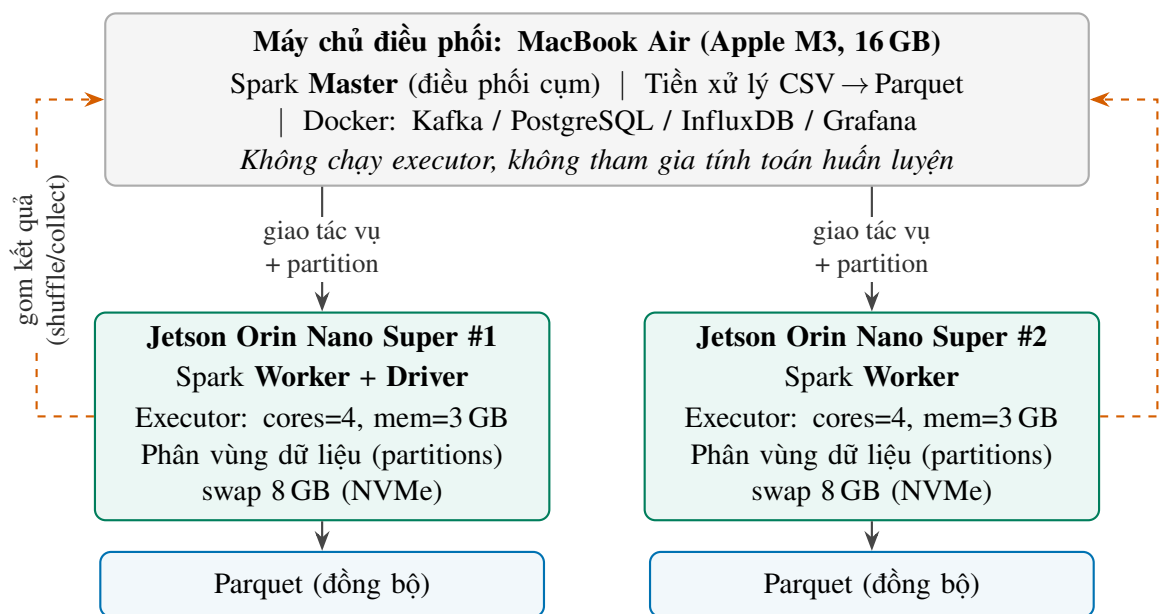
Hình 4.1. Cụm huấn luyện phân tán Apache Spark Standalone: MacBook giữ vai trò master điều phối (không chạy executor ), hai Jetson Orin Nano Super là worker/executor thực thi tính toán; dữ liệu Parquet được phân vùng và đồng bộ sang cả hai nút, kết quả được gom về qua shuffle/collect .
