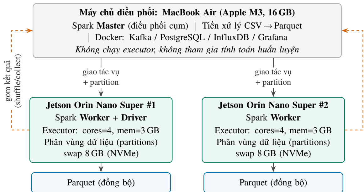
Hình 4.1. Cụm huấn luyện phân tán Apache Spark Standalone: MacBook giữ vai trò master điều phối (không chạy executor), hai Jetson Orin Nano Super là worker/executor thực thi tính toán; dữ liệu Parquet được phân vùng và đồng bộ sang cả hai nút, kết quả được gom về qua shuffle/collect.
