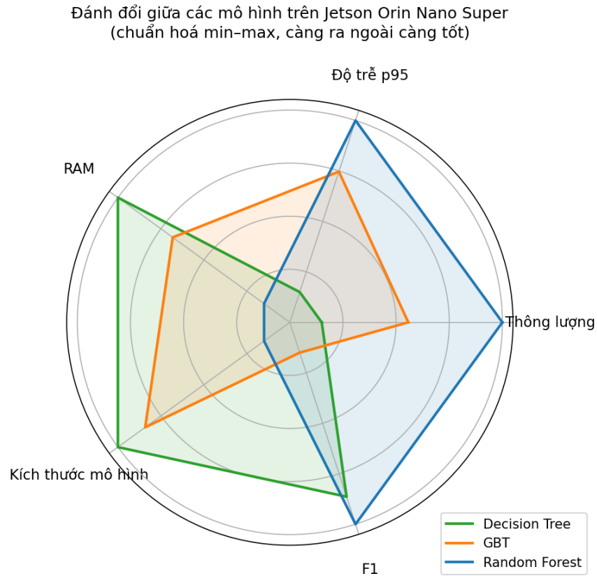
Hình 4.14. Biểu đồ radar thể hiện sự đánh đổi (trade-off) giữa các mô hình trên thiết bị biên
