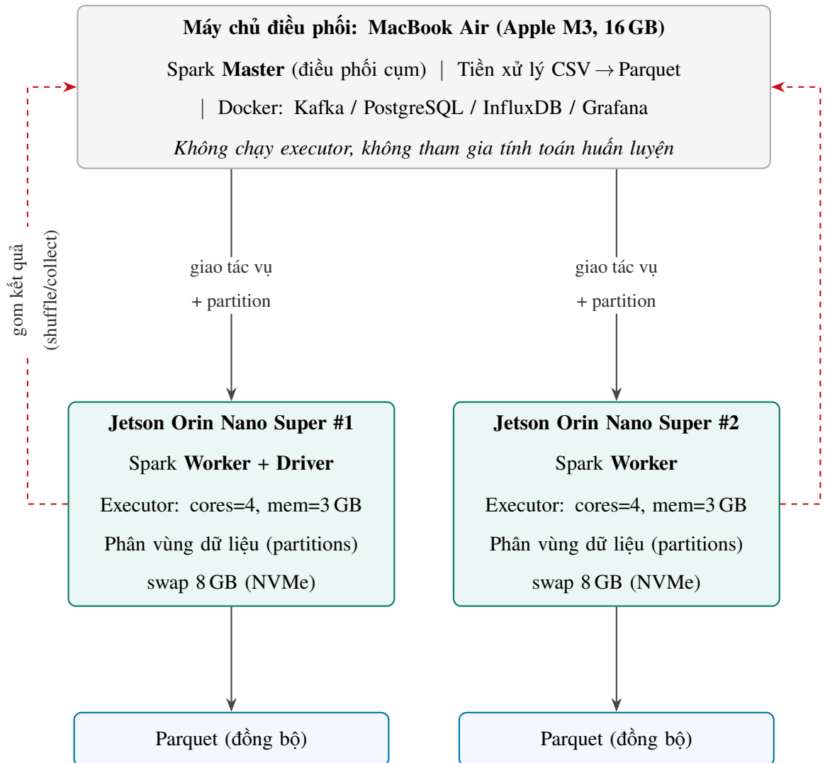
Hình 4.1. Cụm huấn luyện phân tán Apache Spark Standalone: máy chủ điều phối (master) và hai Jetson worker/executor
