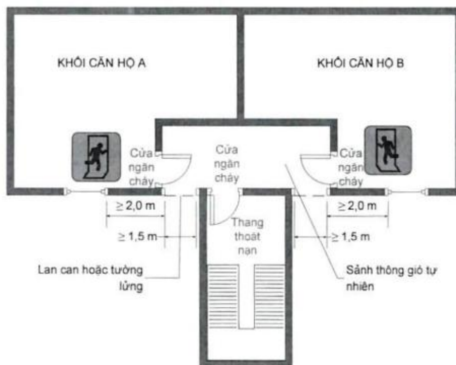
Hình I.8 - Khoảng đệm không nhiễm khói dẫn vào buồng thang bộ loại N1
