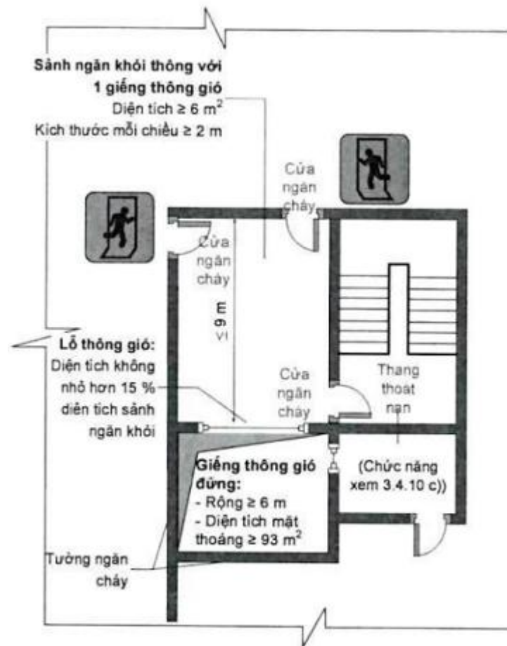
f) Khoảng đệm không nhiễm khói là một sảnh ngăn khói có thông gió tự nhiên qua giếng đứng Hình I.8 (tiếp theo)
