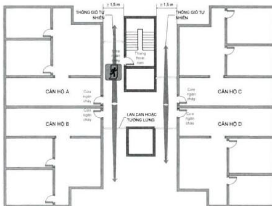
g) Khoảng đệm không nhiễm khói là một sảnh chung nằm giữa các khối nhà và bảo đảm điều kiện lưu thông của không khí qua sảnh nhờ những lỗ thông trên hai tường đối diện
