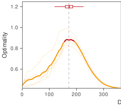
SSP2-4.5
