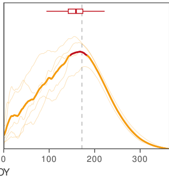
SSP5-8.5
