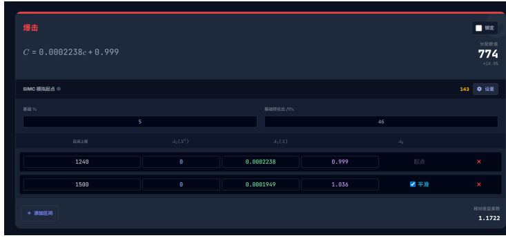
Figure 3: 单项属性配置卡片（以暴击为例）
