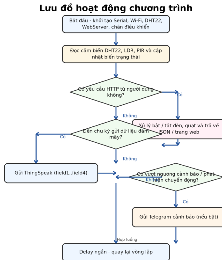
Hình 3.2. Lưu đồ hoạt động của chương trình điều khiển
