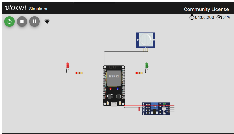
Hình 4.1. Sơ đồ nối dây mô phỏng trên Wokwi (phiên bản chạy cuối)
