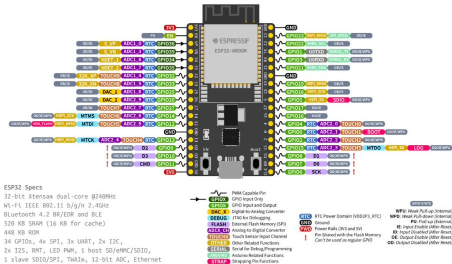
Hình 1: Vi điều khiển ESP32 – DevKitC
