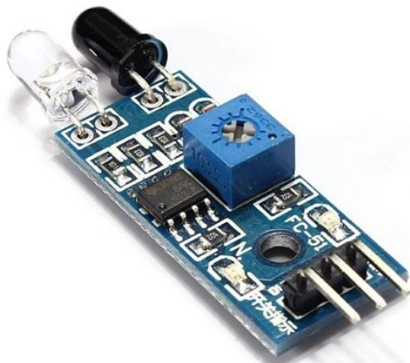
Hình ảnh thực tế của module cảm biến vật cản hồng ngoại FC-51
