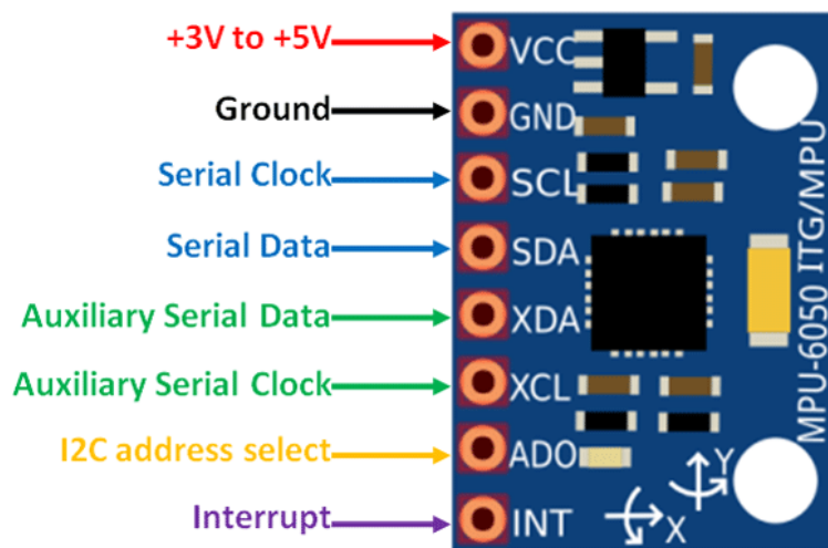
HÌNH 3: SƠ ĐỒ CHÂN MPU6050
