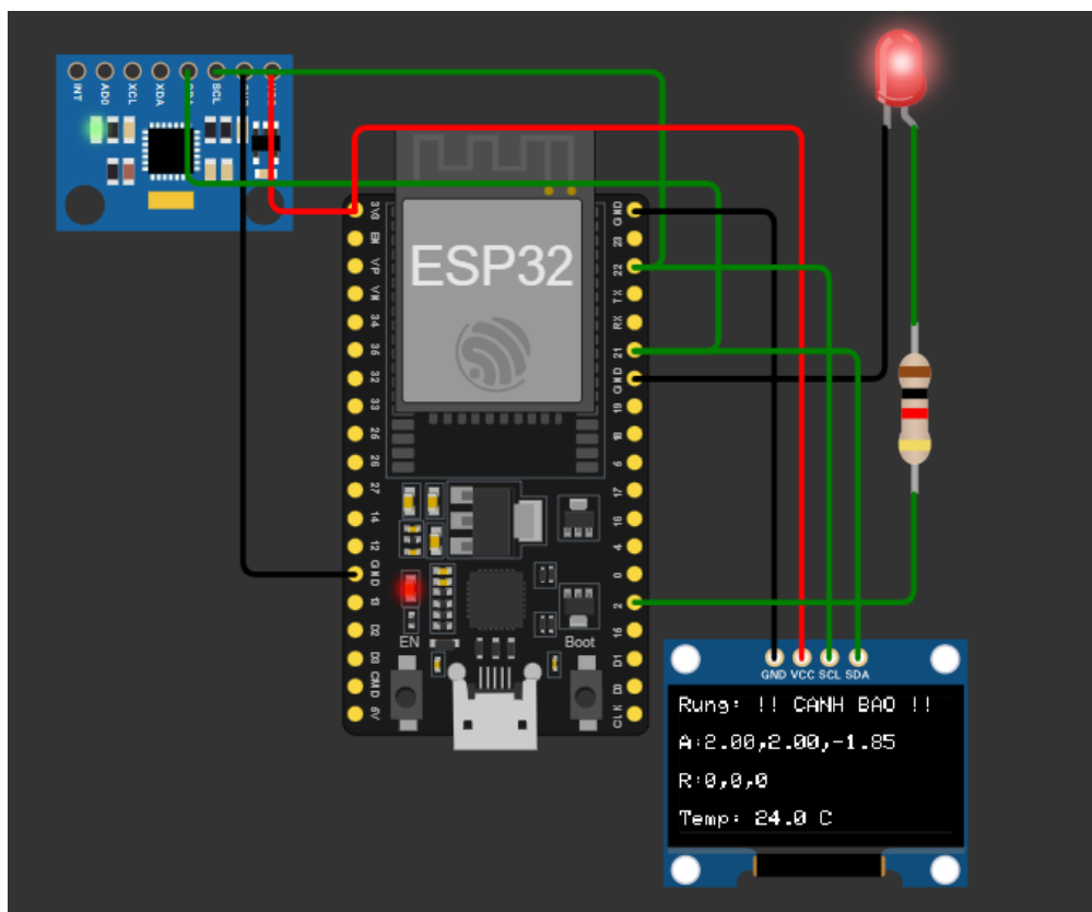
Hình 7: sơ đồ kết nối wokwi.
