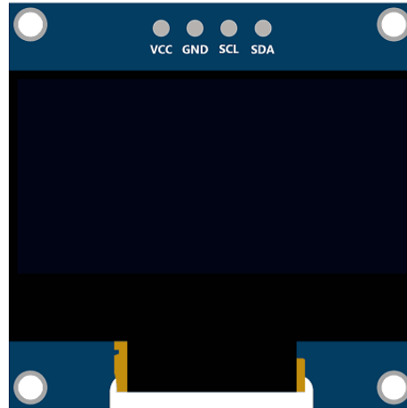
Hình 6. Chân cắm màn hình OLED
