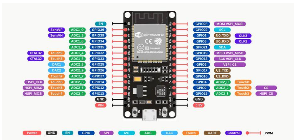
Hình 1: sơ đồ chân ESP32.
