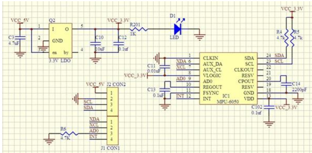
Hình 4 : sơ đồ kết nối MPU6050
