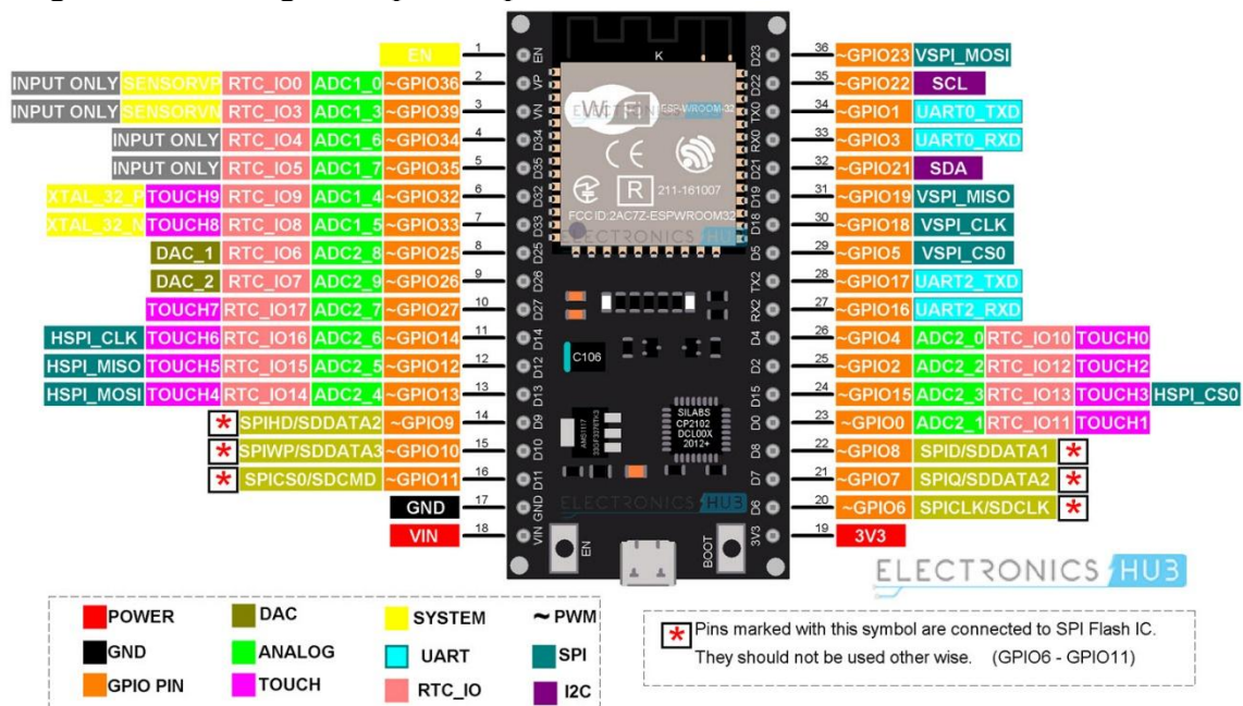
Hình 2.1: Sơ đồ chân và các cổng kết nối của vi điều khiển ESP32
