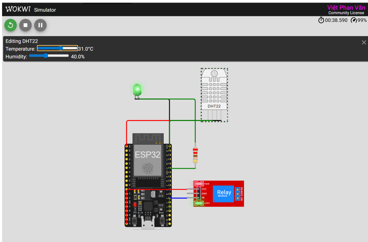
Hình 4.2.2. Hệ thống khi nhiệt độ 31°C (quạt bật, LED sáng)
