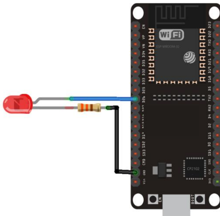
Hình 2.3: Đèn LED
