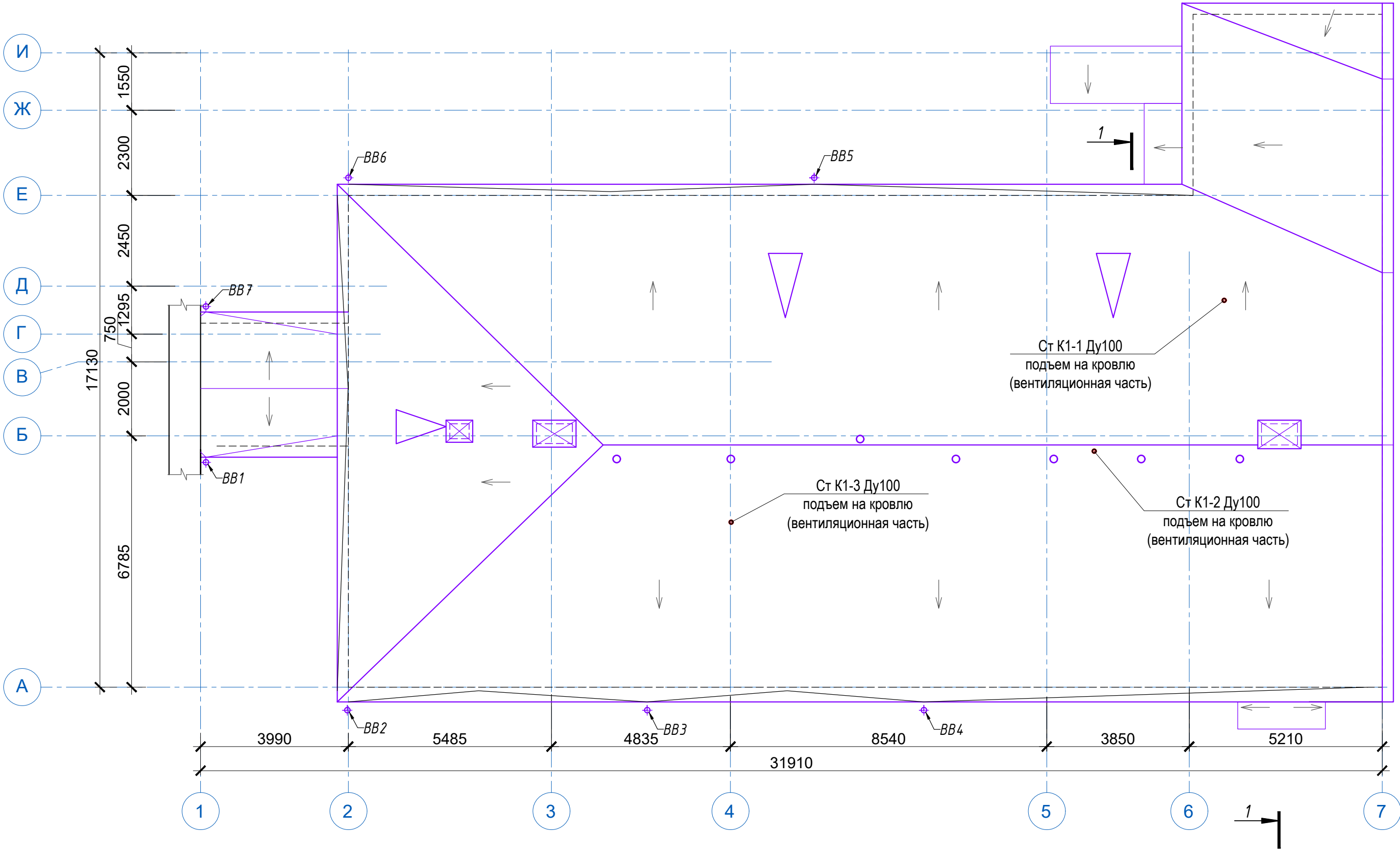
План кровли М 1:100
