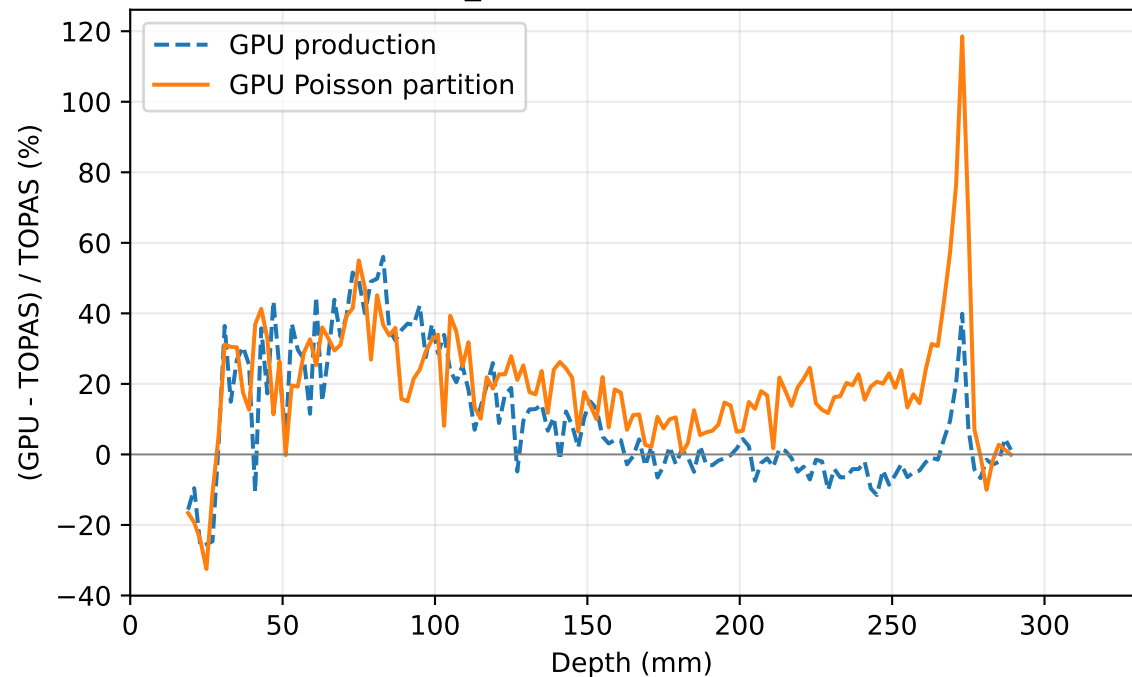
b1_400 halo relative error
