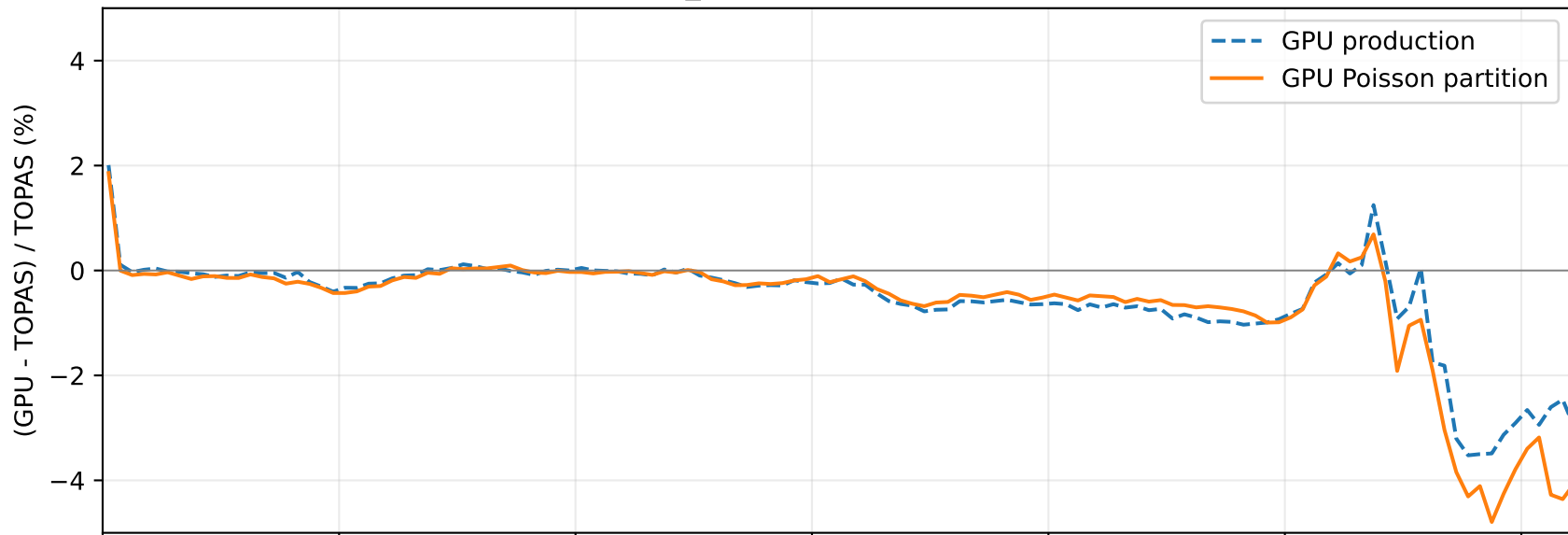
b2_150 IDD relative error
