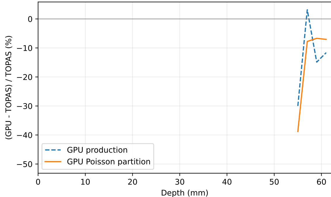
b2_150 halo relative error
