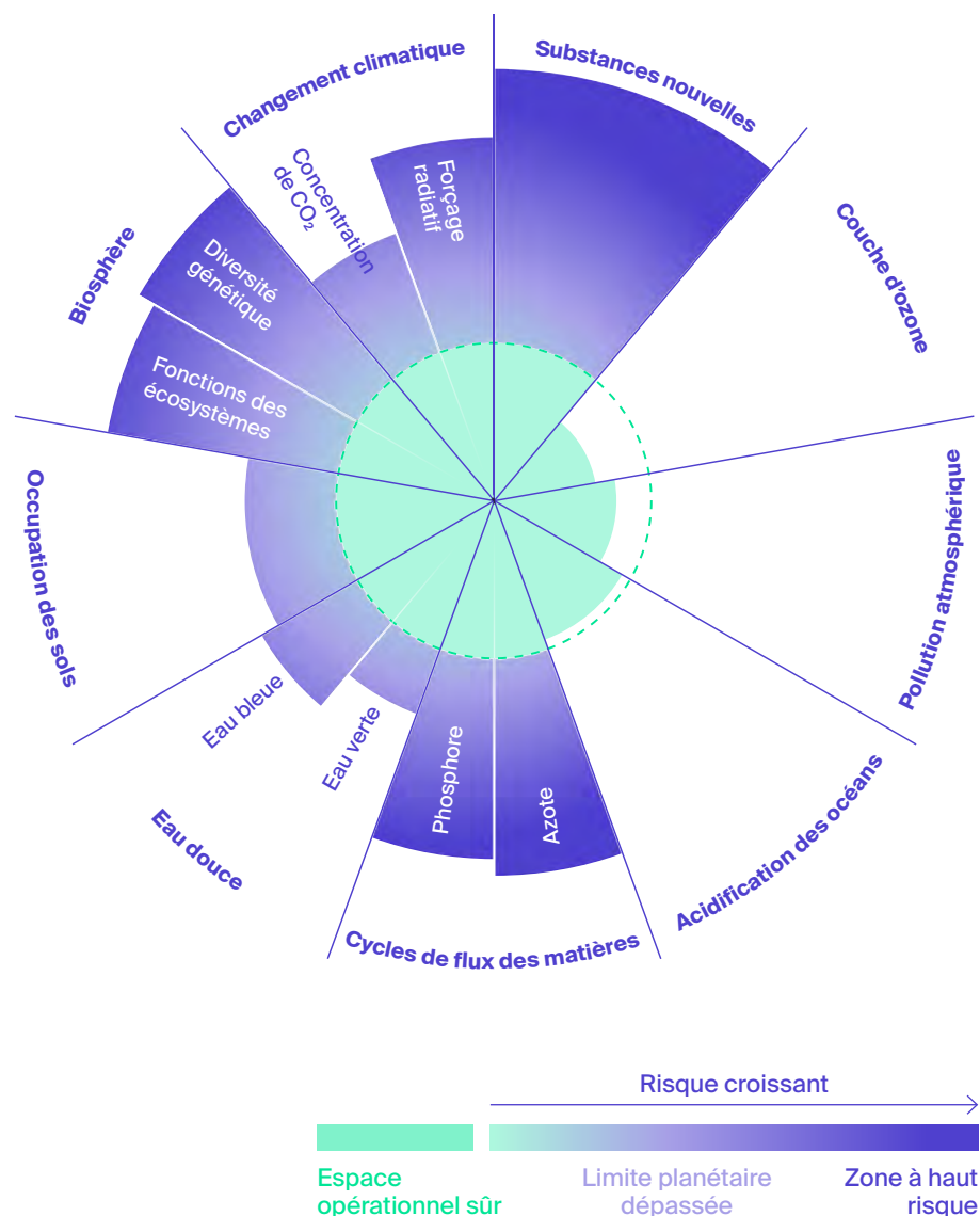
Fig. 5 Les neuf limites planétaires. Graphique adapté d'après Richardson et al., 2023.
