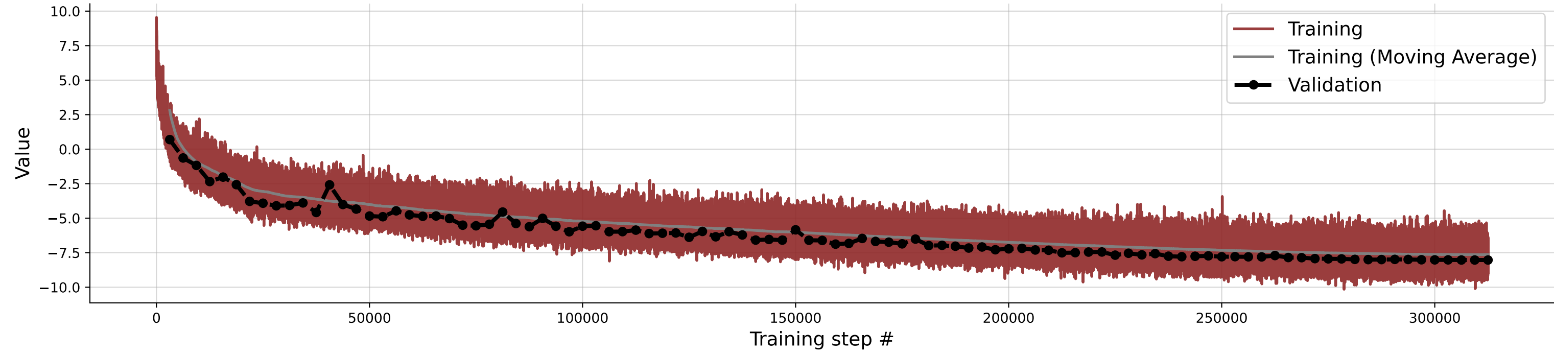
W.Decay
